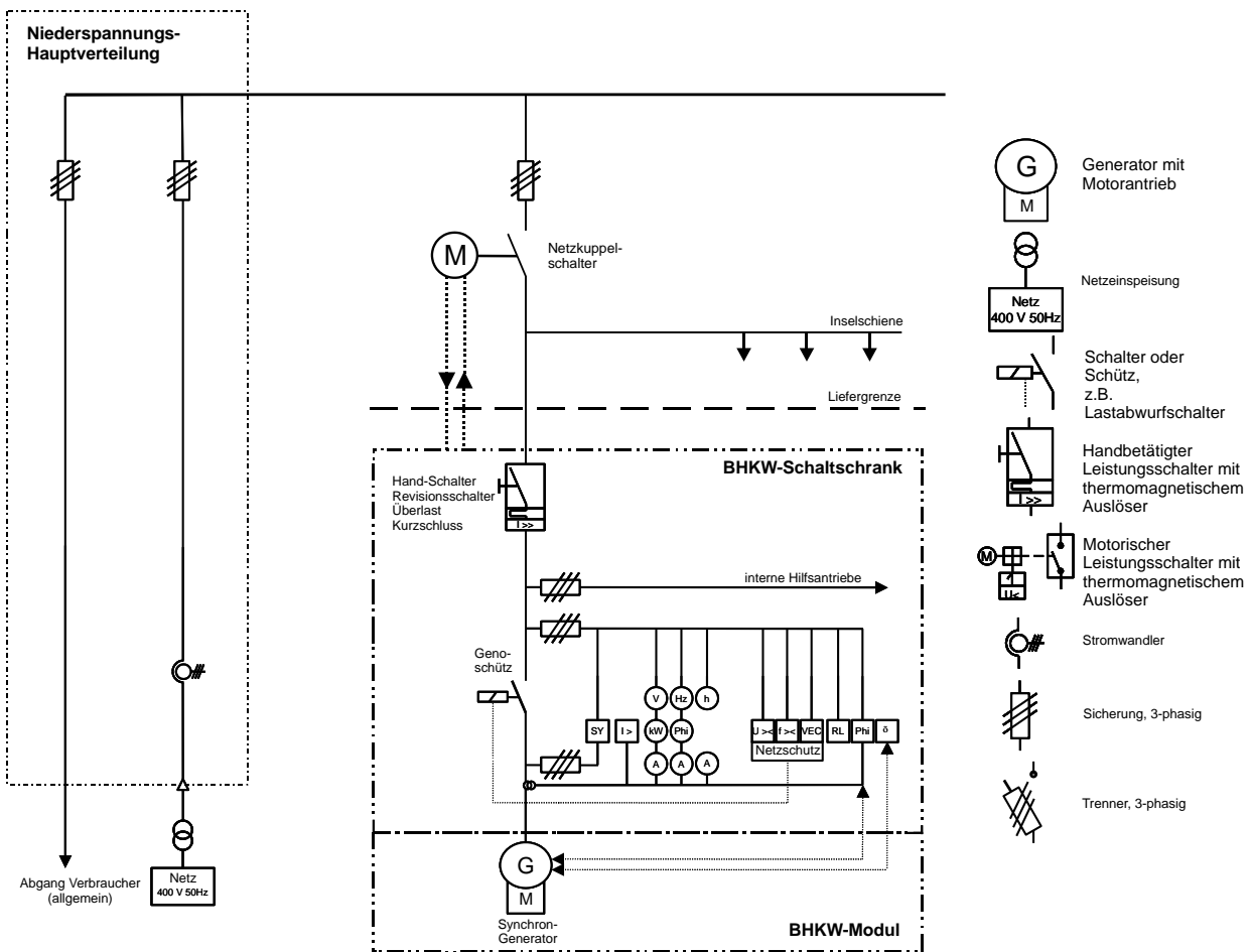
Abb. 6 Prinzipschaltbild der elektrischen Einbindung eines BHKW im Inselbetrieb
