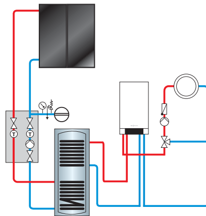
Solare Trinkwassererwärmung
