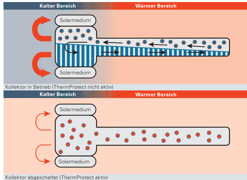
Die selbstregelnde Heatpipe der Vakuum-Röhrenkollektoren Vitosol 300-TM und Vitosol 200-TM: Bei Erreichen der Grenztemperatur von ca. 120 °C kann das Medium nicht mehr kondensieren, dadurch ist der Wärmetransport unterbrochen und die Anlage damit gegen zu hohe Stagnationstemperaturen geschützt.
