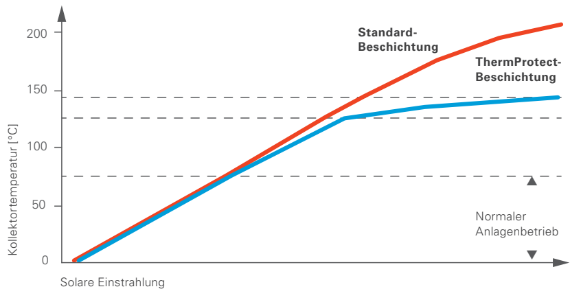
Im regulären Kollektorbetrieb verhält sich die ThermProtect-Beschichtung der Flachkollektoren wie eine herkömmliche Absorberbeschichtung. Oberhalb von 75 °C Kollektortemperatur erhöht sich die Abstrahlung um ein Vielfaches und verhindert im Stagnationsfall zuverlässig die Überhitzung und Dampfbildung.
